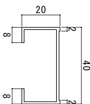
面格子横材
