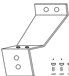
壁付金具
