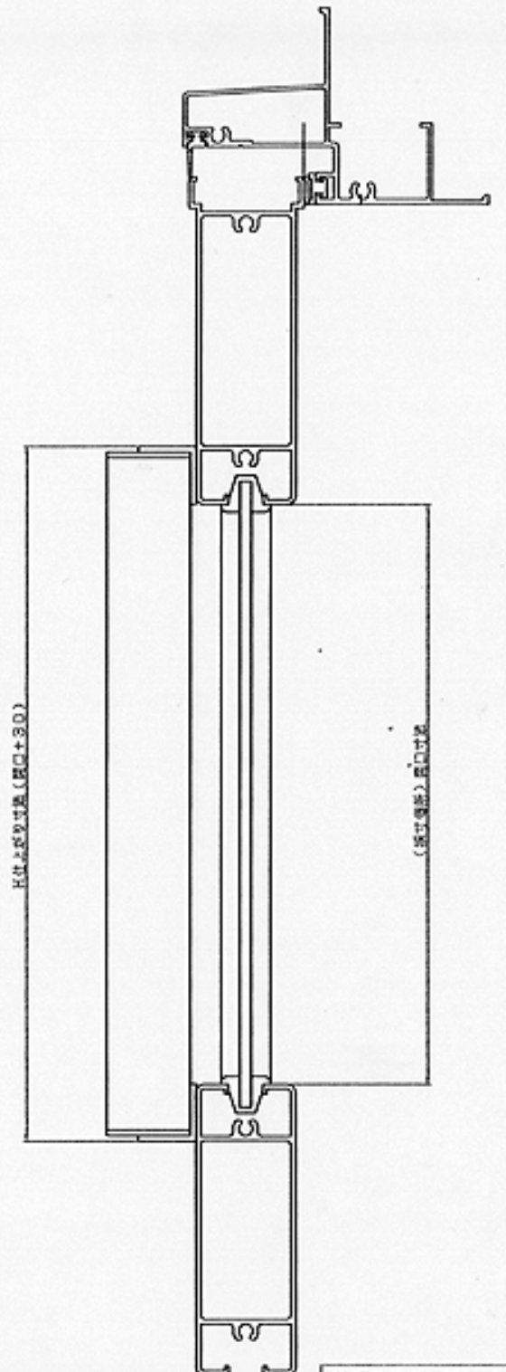
勝手口格子シアングル納まり
