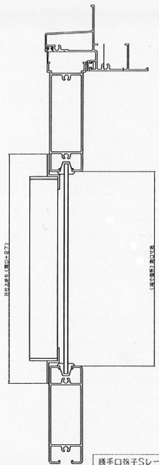
勝手口格子Sレール納まり
